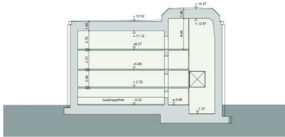
Schnitt C-D
